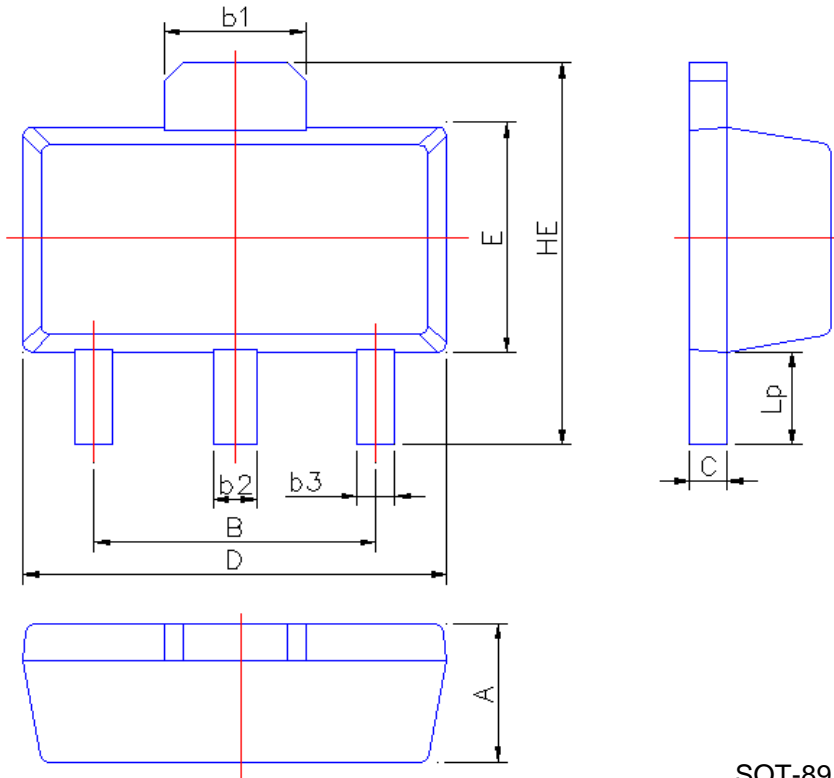
SOT-89 1.0
