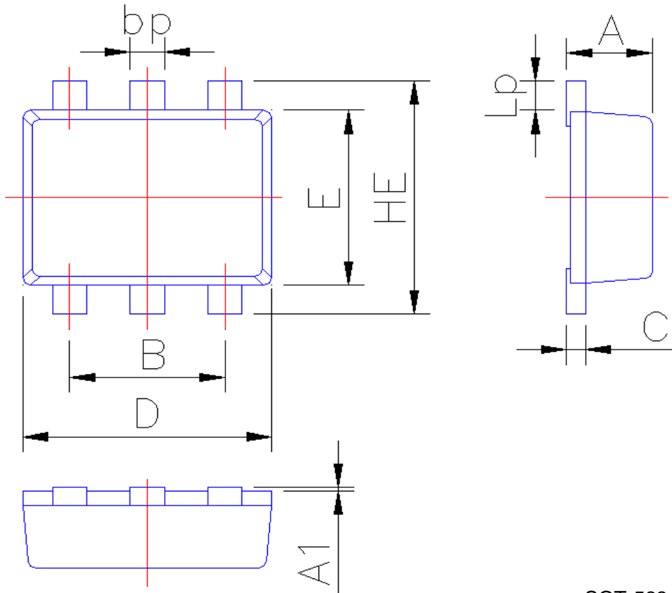
SOT-563 1.0
