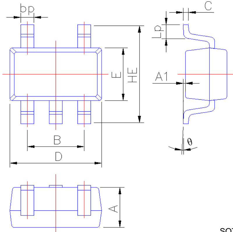
SOT-353 1.0
