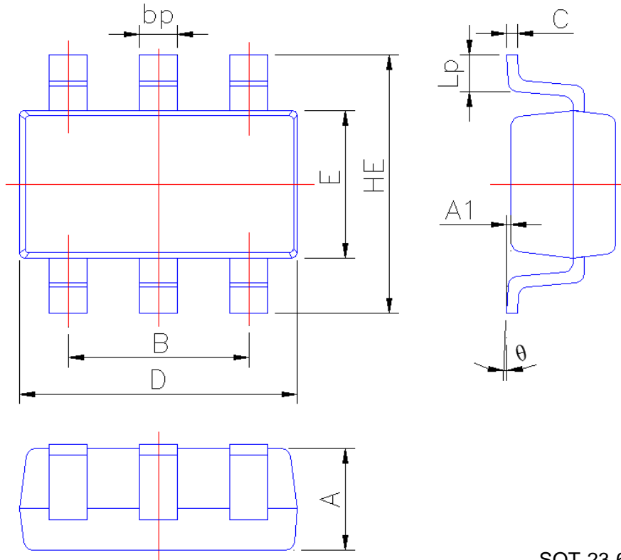
SOT-23-6L 1.0
