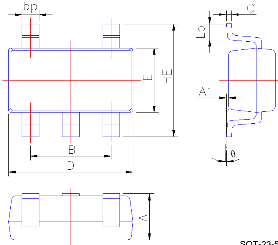
SOT-23-5L 1.0
