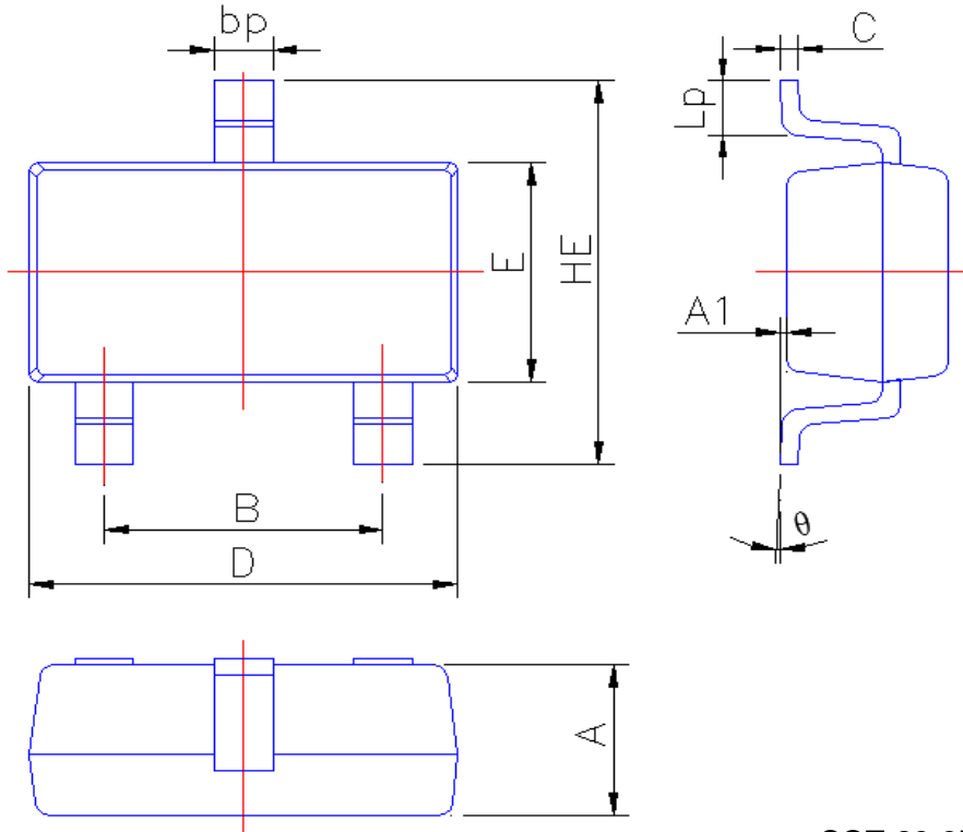
SOT-23-3L 1.0
